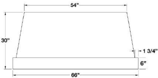
66" Dimensions
