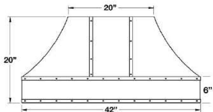
42" Dimensions
