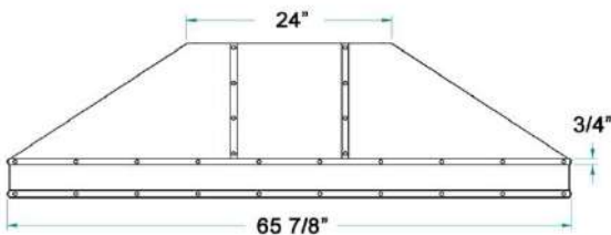
66" Dimensions
