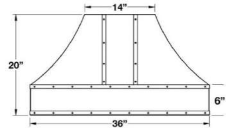
36" Dimensions
