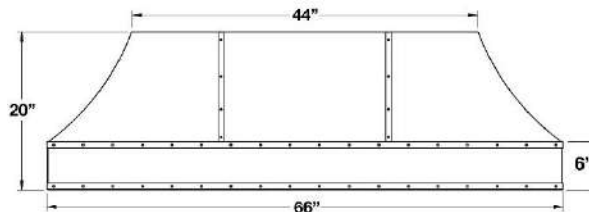
66" Dimensions
