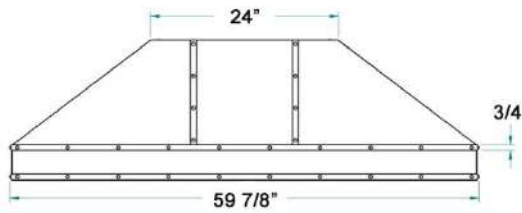
60" Dimensions
