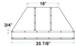
36" Dimensions
