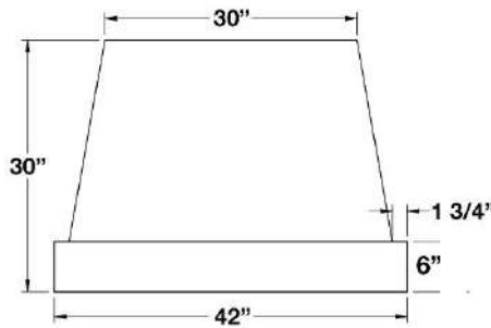
42" Dimensions
