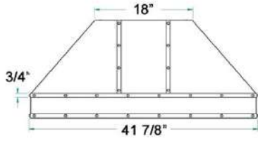
42" Dimensions
