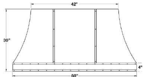
60" Dimensions
