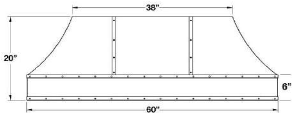
60" Dimensions
