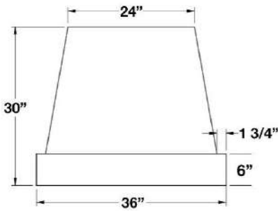
36" Dimensions
