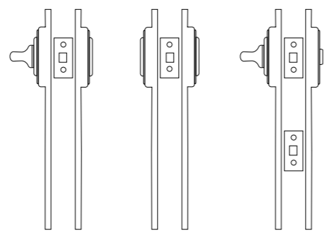
103 EP 104 EP 106 EP
