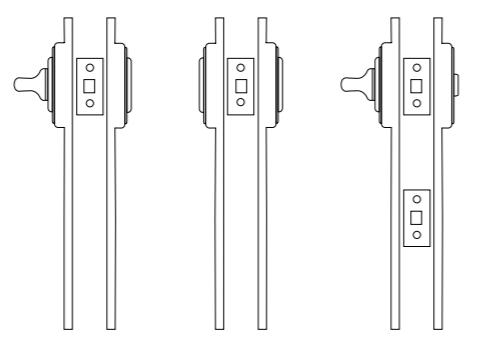
103 ET 104 ET 106 ET
