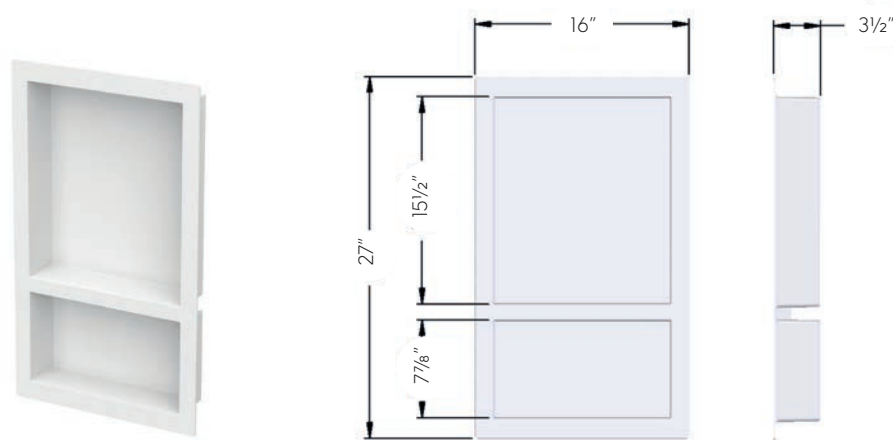
FastNICHE Double
