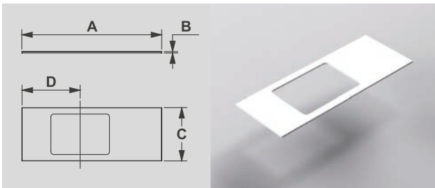
A: 1205 mm B: 12 mm C: 460 mm D: 500 mm
