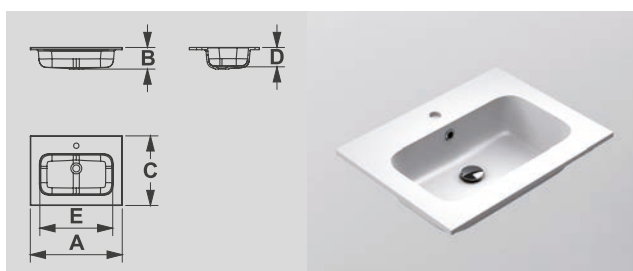
A: 605 mm B: 143 mm C: 460 mm D: 128 mm E: 480 mm
