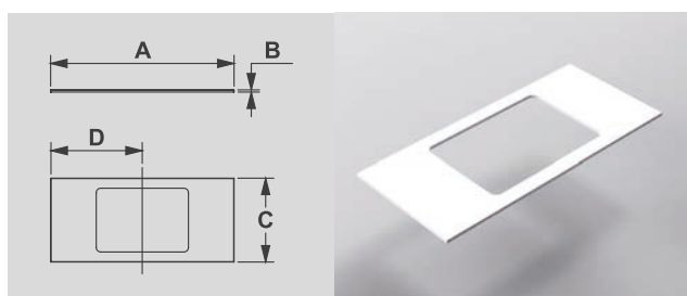
A: 1005 mm B: 12 mm C: 460 mm D: 1005 mm
