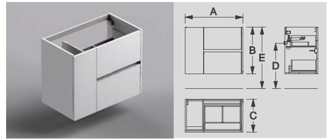
A: 800 mm B: 650 mm C: 458 mm D: 240-600 mm E: 855 mm
