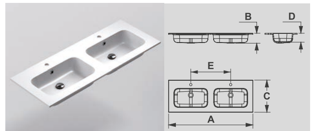
A: 1205 mm B: 143 mm C: 460 mm D: 128 mm E: 570 mm
