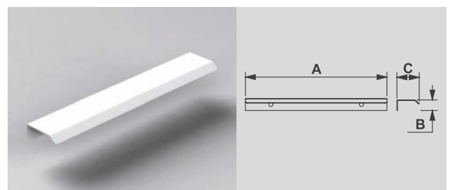
A: 198 mm B: 7 mm C: 20 mm
