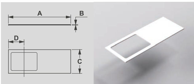
A: 1205 mm B: 12 mm C: 460 mm
