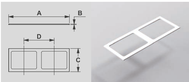
A: 1205 mm B: 12 mm C: 460 mm D: 600 mm
