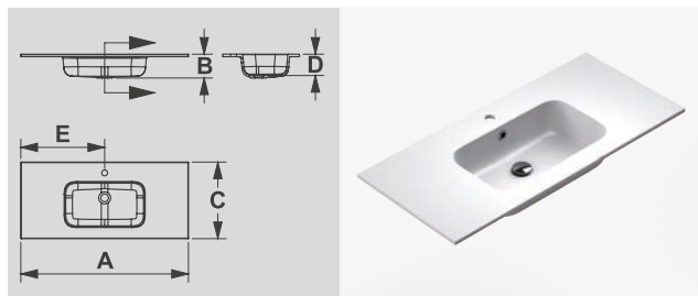
A: 1005 mm B: 143 mm C: 460 mm D: 128 mm E: 500 mm
