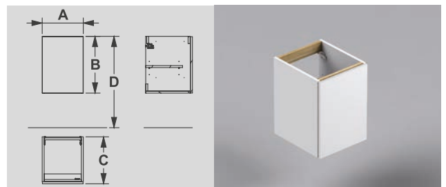
A: 400 mm B: 550 mm C: 458 mm D: 885 mm
