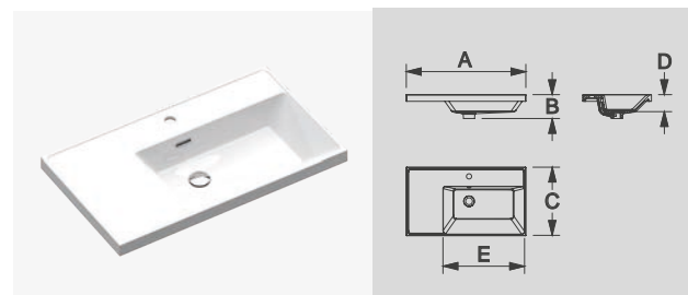
A: 806 mm B: 161 mm C: 463 mm D: 115 mm E: 546 mm
