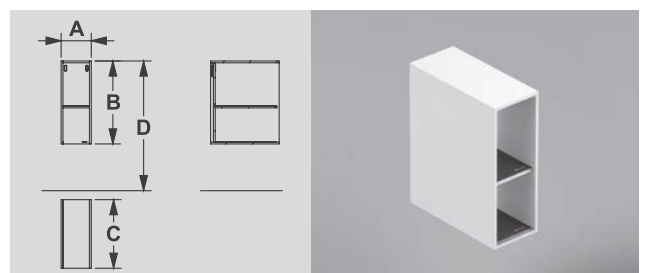
A: 200 mm B: 550 mm C: 458 mm D: 885 mm
